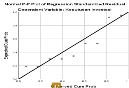
Gambar 1. Uji Normalitas
