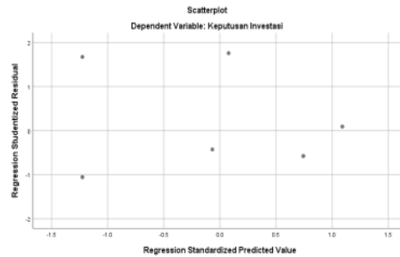
Gambar 2. Uji Heterokedastisitas
