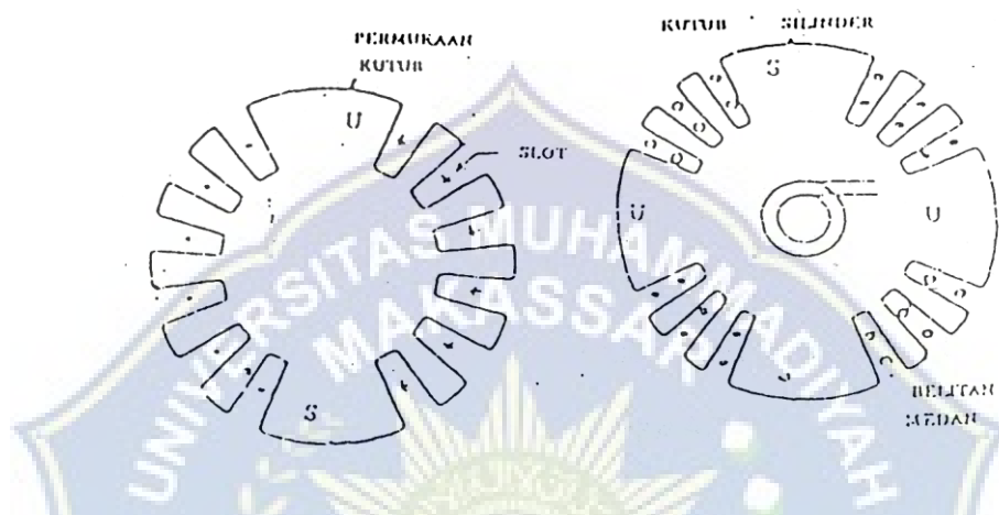
Gambar 2.9 Penampang rotor untuk jenis kutub silinder
