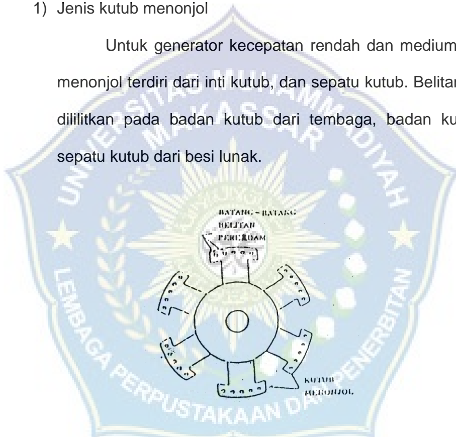
Gambar 2.8 Penampang rotor untuk jenis kutub menonjol dengan belitan peredam
