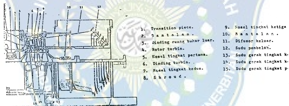
Gambar 4.7 Konstruksi Turbin
