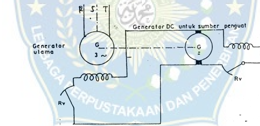
Gambar 2.10 Generator dengan penguat generator shunt
