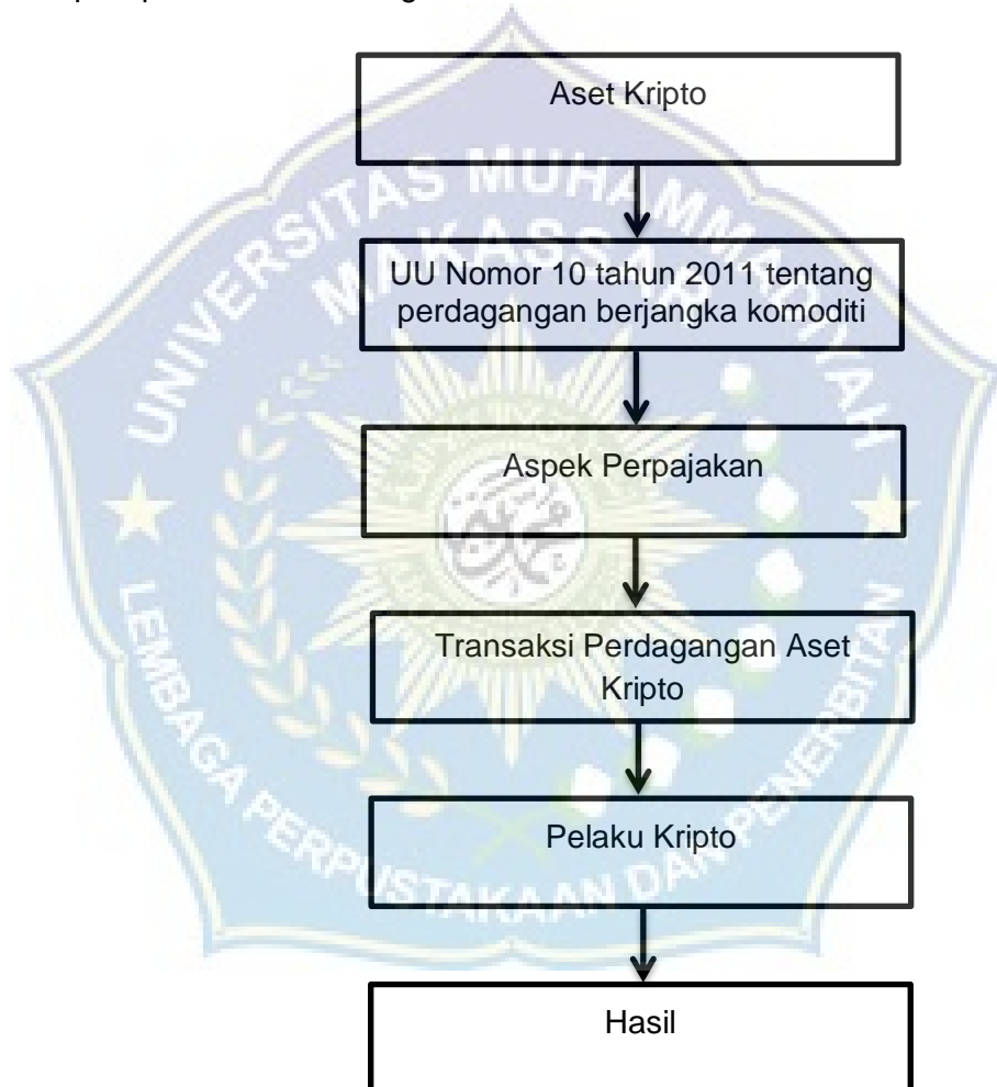
Gambar 2. 1 Kerangka Berpikir
