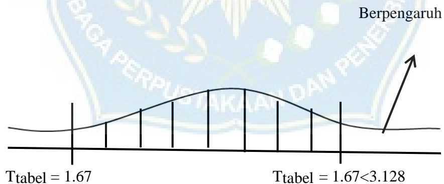
Gambar 1.4 : Kurva pengujian dua sisi
