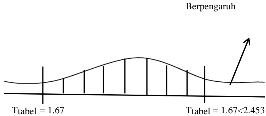
Gambar 1.3 : Kurva pengujian dua sisi
