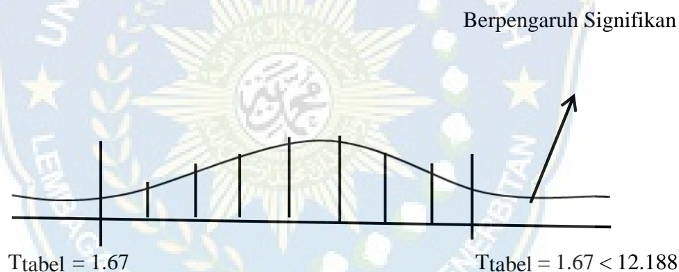
Gambar 1.2 : Kurva pengujian dua sisi
