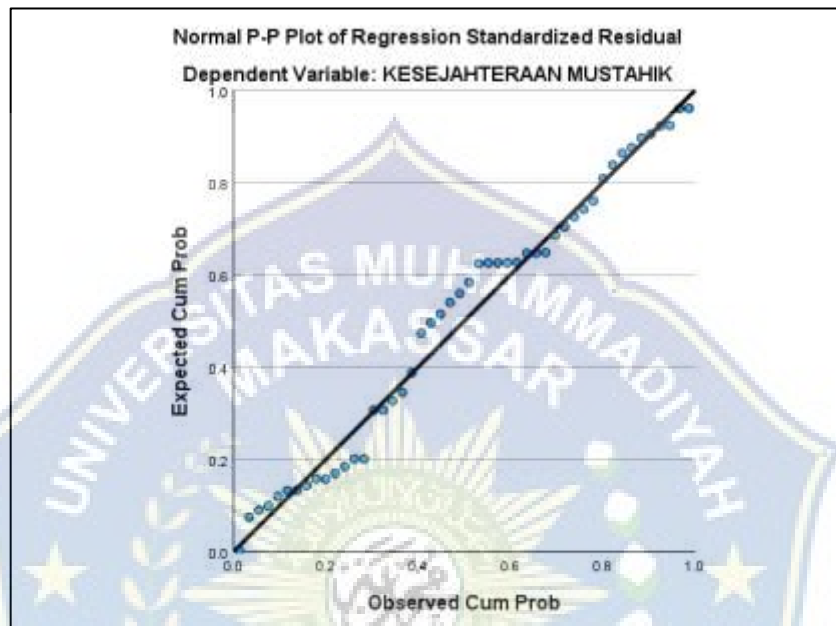
Gambar 4.2 Hasil Uji Grafik Normal P- Plot (Sumber: Hasil Olah Data, 2024)
