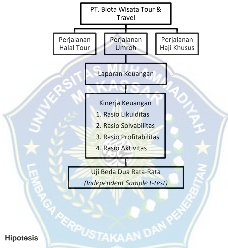
Gambar 2. 1 Kerangka Pikir
