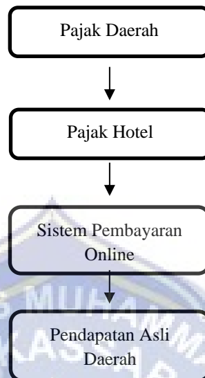
Gambar 2.1 Kerangka Konseptual
