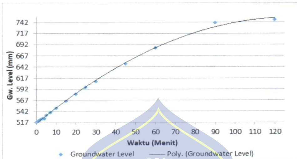
Gambar 12. Grafik Hubungan Waktu Hujan VS Fluktuasi Muka Air Tanah (Hujan Kelima)
