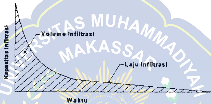
Gambar 3. Kurva Infiltrasi (Bambang Triatmodjo, 2008)
