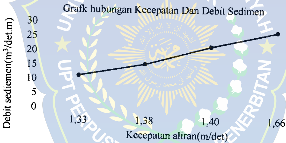
Gambar 14. Grafik hubungan Grafik hubungan Kecepatan Dan Debit Sedimen
