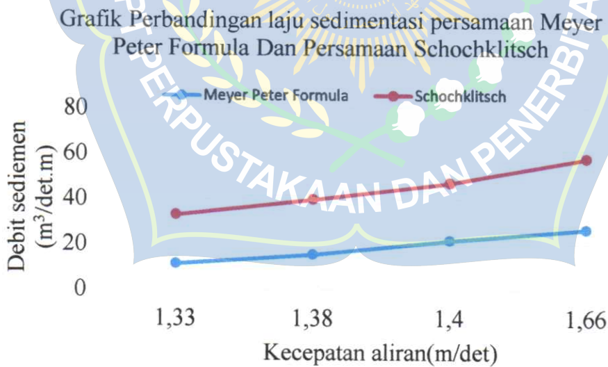
Gambar 19. Grafik Perbandingan laju sedimentasi persamaan Meyer Peter Formula Dan Persamaan Schochklitsch
