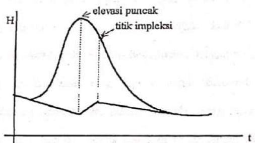
Gambar 7.2: Pemisahan Aliran Dasar Dengan Variable Slope Method (Sri Harto, 1993)
