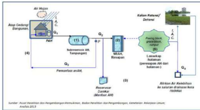
Gambar 2.7: Pengelolaan Drainase Perkotaan Secara Terpadu Berwawasan Lingkungan (Ecodrain) (Balitbang Kementerian PU, 2013)
