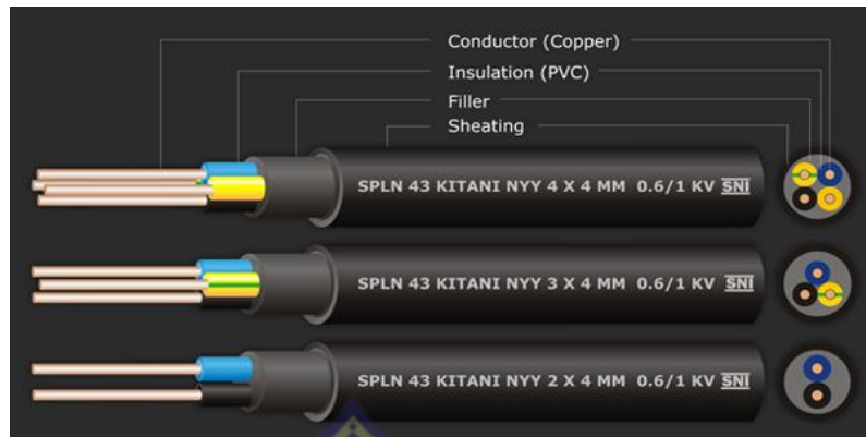
Gambar 2.3 Kabel NYY
