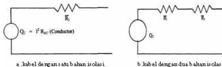
Gambar 2.9 Rangkaian termal untuk kabel dengan satu sumber kalor.
