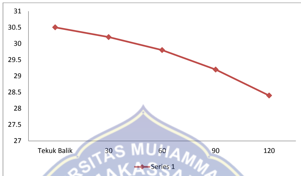
Gambar 4.2 Pengaruh sudut penekukan terhadap temperatur pada isolasi dengan arus 1.7A
